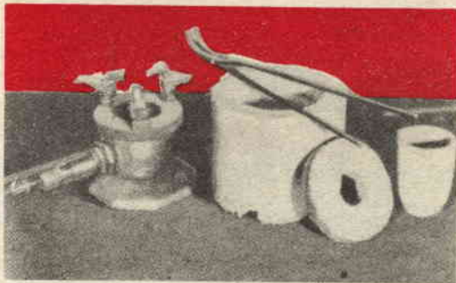
Il bruciatore, la camicia termoisolante, il coperchio ed il crogiuolo sono qui visibili. Il corpo della fornace è un giunto a T da mm. 30x30x50; le aperture rettangolari laterali, che possono essere chiuse dal clip rotante di ottone servono per la regolazione di afflusso di aria di carburazione
