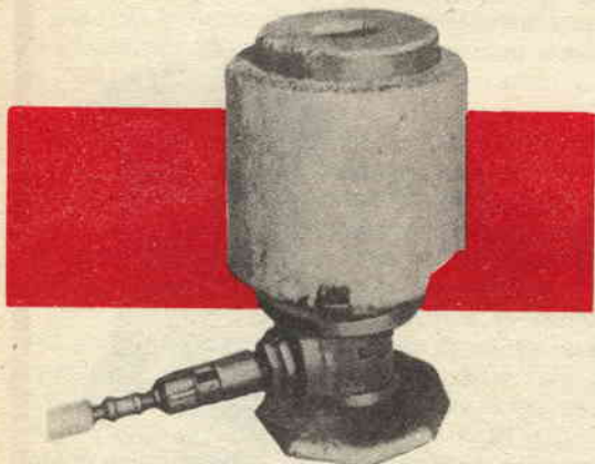
Con la fornace descritta è molto facile realizzare delle gettate in alluminio di qualche centinaio di grammi, come anche delle colate più piccole in numero maggiore
